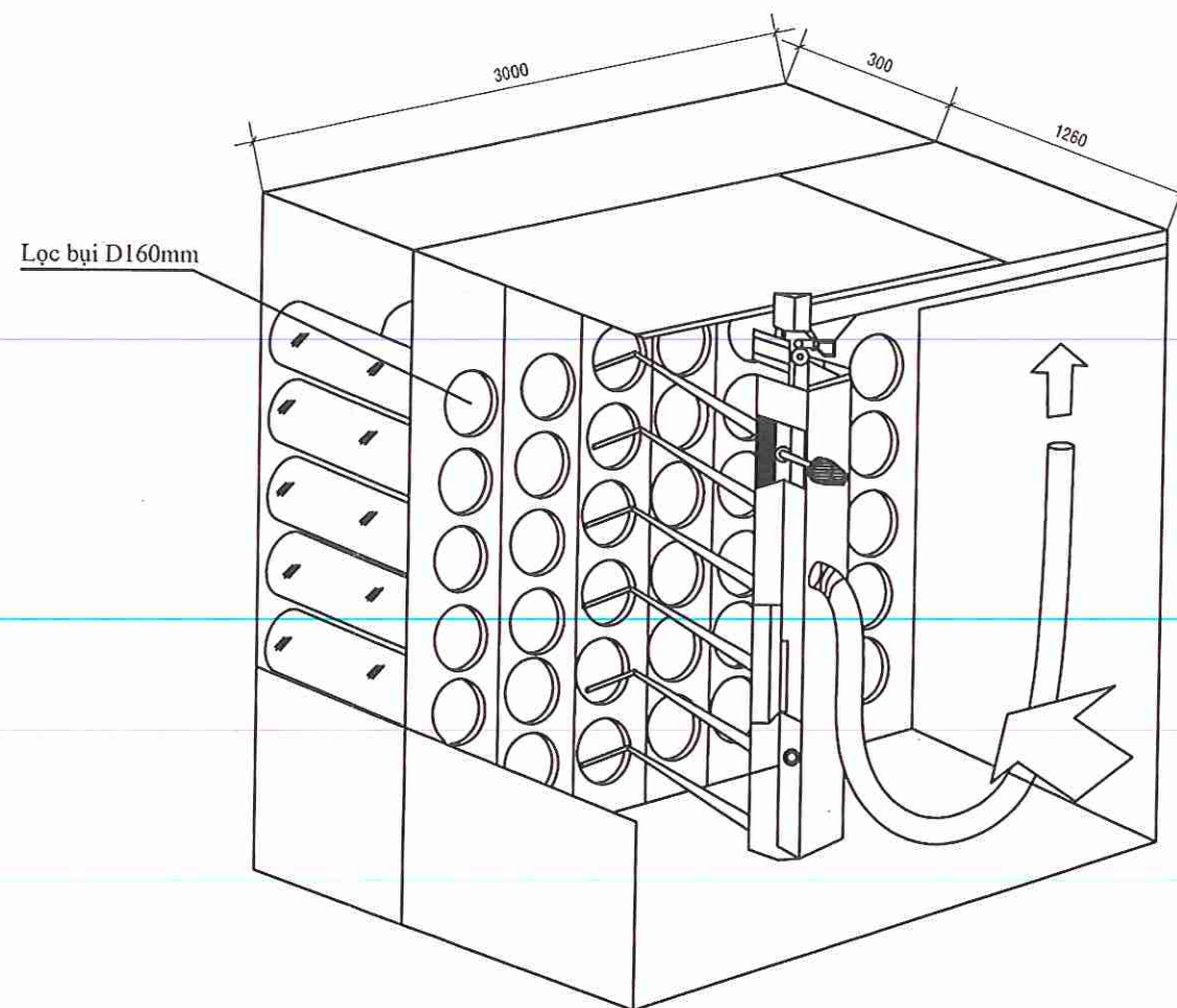
HỆ THỐNG LỌC BỤI TỔ ONG
