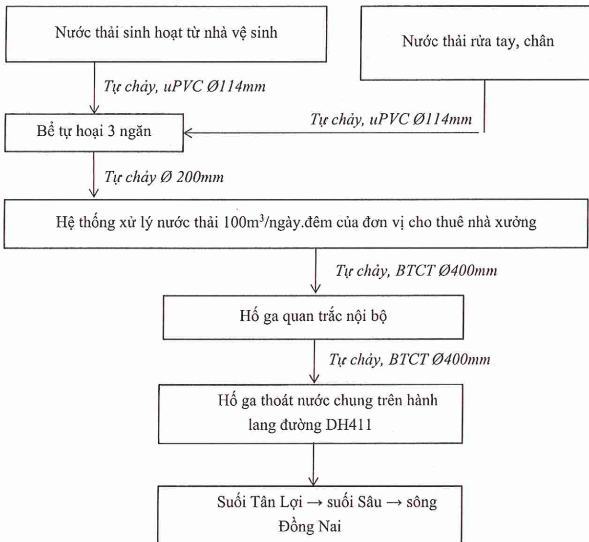
Hình 4. 7. Sơ đồ thu gom, thoát nước thải của dự án
