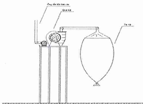
Hình 4. 6. Cấu tạo lọc bụi túi vải
