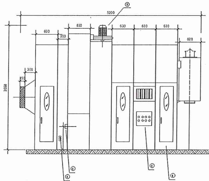
Hình 4. 5. Cấu tạo thiết bị lọc bụi dạng tổ ong
