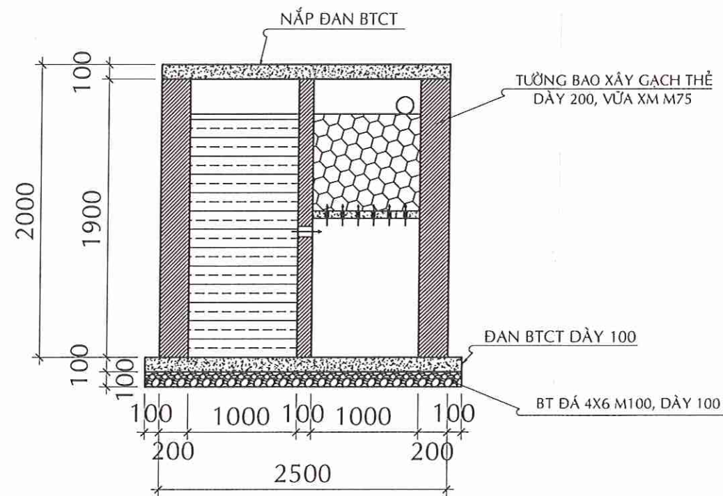
MẶT CẮT B-B TL 1/50
