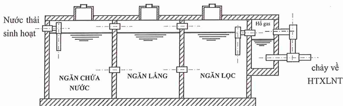
Hình 4. 8. Cấu tạo bể tự hoại 3 ngăn
