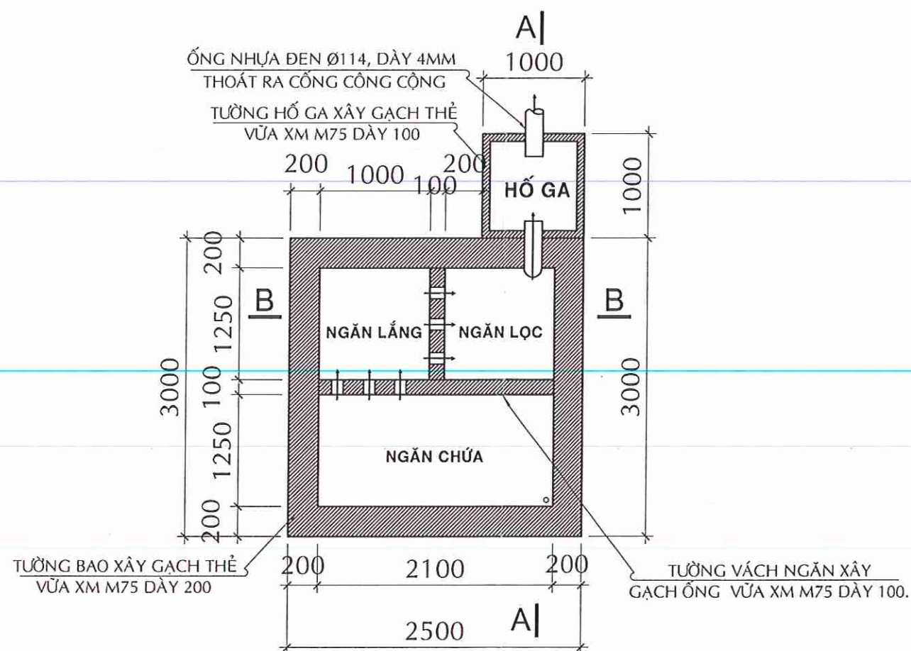
MẶT BẰNG HẦM TỰ HOẠI 1 TL 1/50
