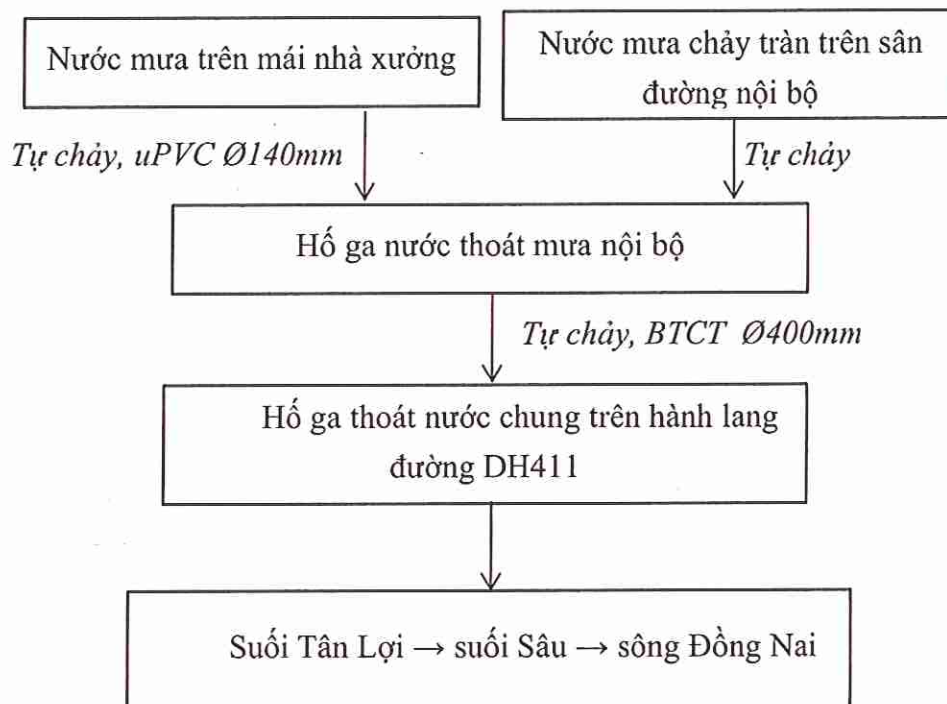
Hình 4. 9. Sơ đồ hệ thống thu gom và thoát nước mưa của dự án trong giai đoạn lắp đặt máy móc, thiết bị
