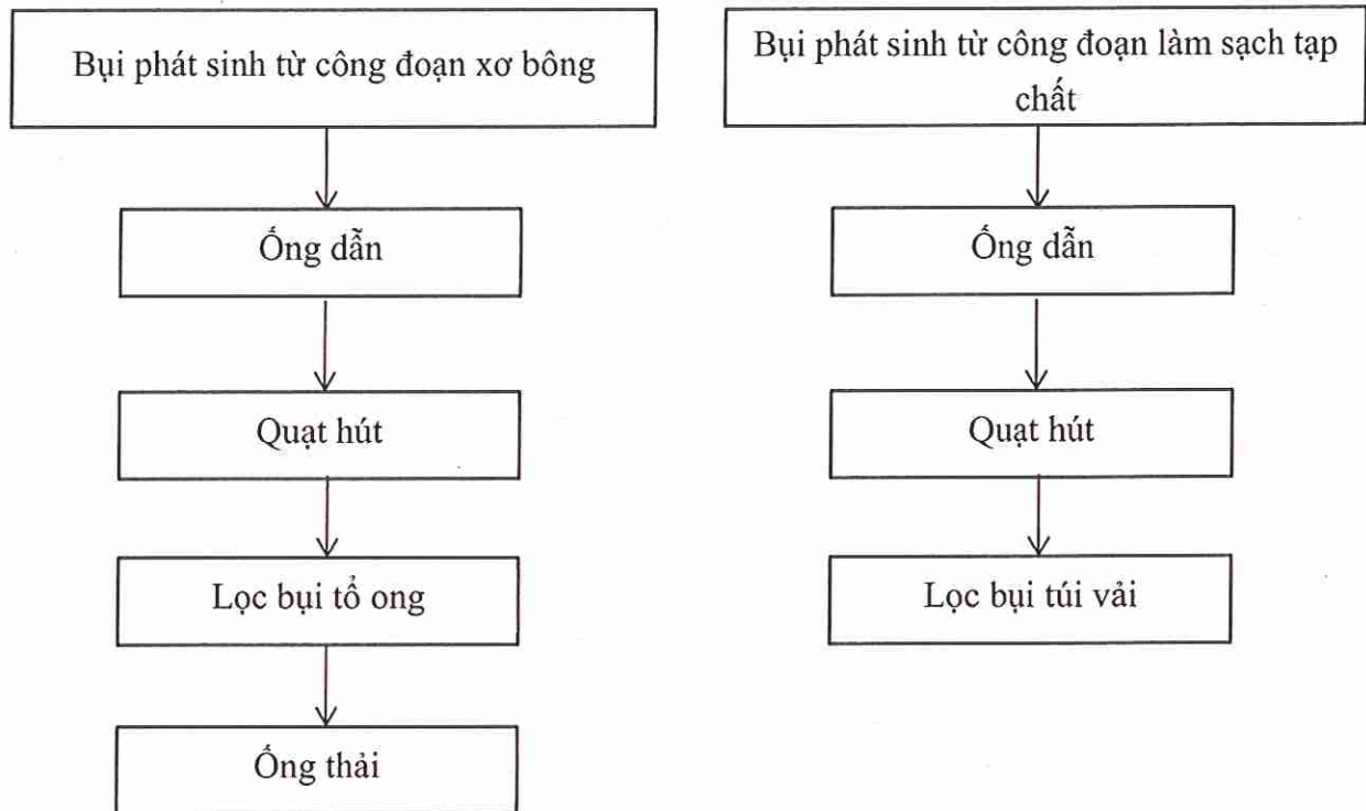
Hình 4. 4. Quy trình thu gom và xử lý khí thải tại xưởng 2 của dự án
